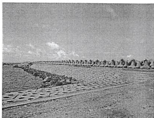
Công trình Kè chống sạt lở Đảo Phú Quý
